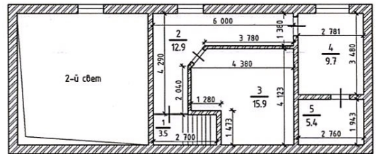
ПЛАН ПОДВАЛА ПОСЛЕ ПЕРЕПЛАНИРОВКИ. М 1:100
