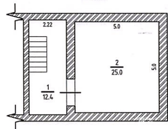
ПЛАН ПОДВАЛА ПОСЛЕ ПЕРЕПЛАНИРОВКИ. М 1:100
