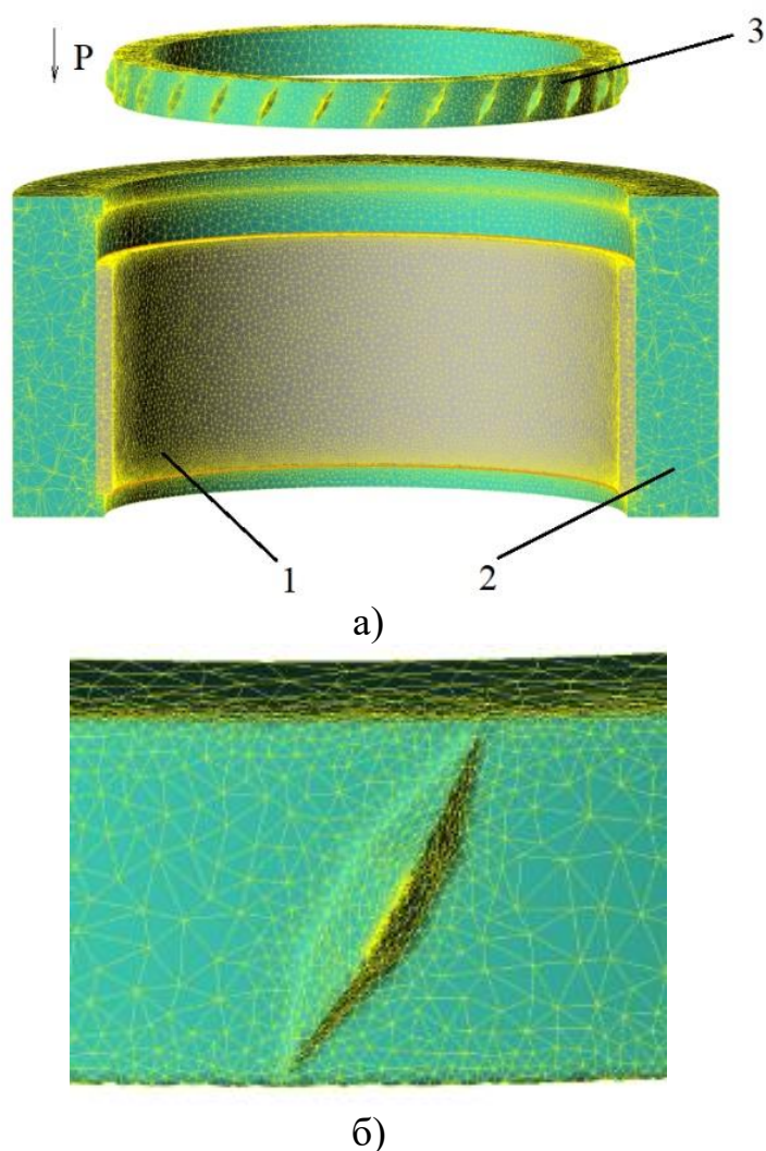
Рисунок 2.3 – Трехмерная модель оснастки (а) с разбиением на конечные элементы для изготовления рифлей на внутренней поверхности металлической оболочки: 1 – заготовка, 2 – контейнер, 3 – рабочая оправка; б – изображения клинового спирального выступа укрупненно
