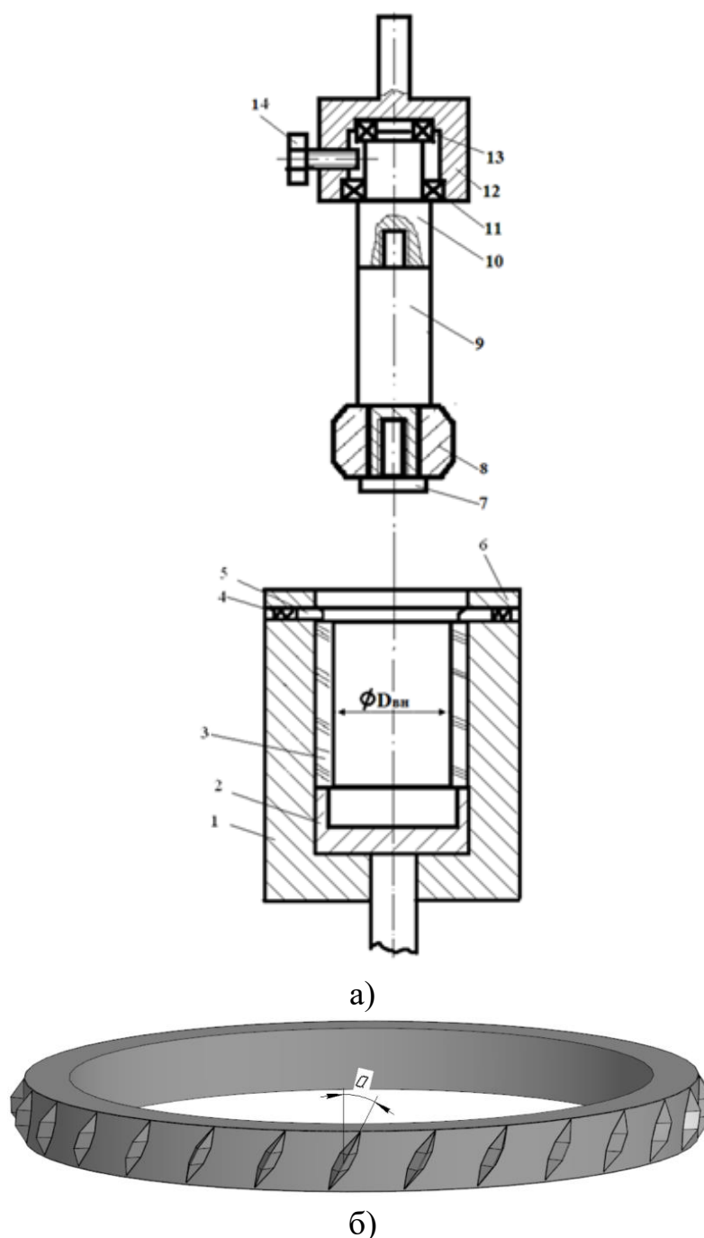
Рисунок 2.2 – Эскиз устройства (а) для реализации локального пластического деформирования и нанесения рифлей на внутренней поверхности оболочки, модель рабочей оправки (б): 1 – корпус, 2 – выталкиватель, 3 – цилиндрическая оболочка (заготовка), 4 – пружины, 5 – съемник, 6 – крышка, 7 – крышка, 8 – рабочая оправка, 9 – инструментальный стержень, 10 – подпятник, 11 – подшипник, 12 – хвостовик, 13 – подшипник, 14 – стопорный винт
