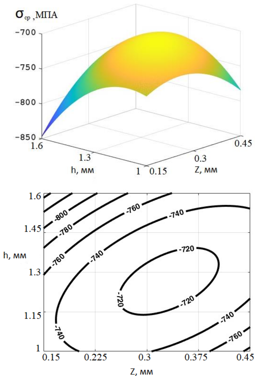
Рисунок 2.32 – Зависимость сжимающих напряжений ( \sigma_{cp} ) от величин ( Z , h )
