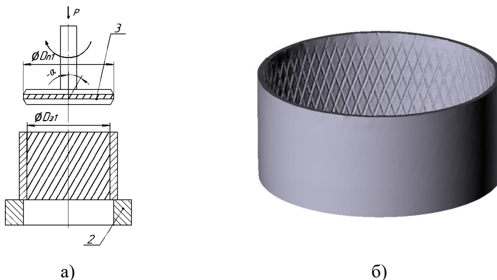
Рисунок 4.3 – Вторая операция для формирования сетки рифлей с раздачей: а – схема процесса, б – полуфабрикат
