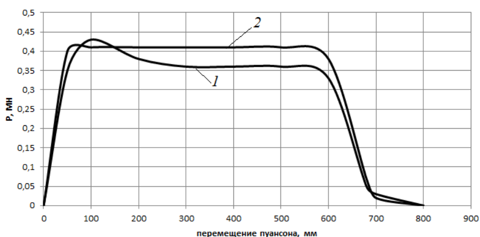
Рисунок 1.15 – Сила после первой операции редуцирования: 1 – экспериментальная кривая; 2 – теоретическая кривая
