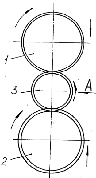
Рисунок 1.5 – Схема процесса: 1 и 2 – ролики, 3 – заготовка
