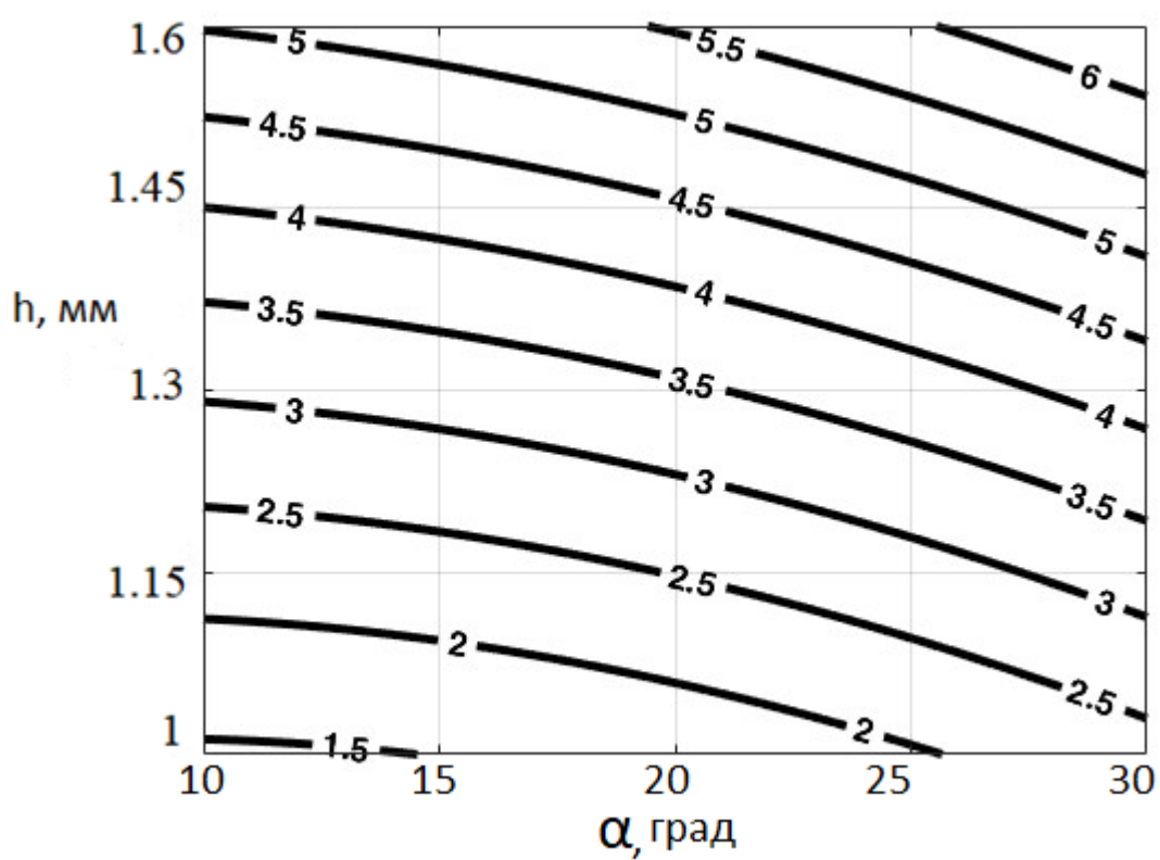
Рисунок 2.15 – Зависимость силы rifления на один выступ ( P_B ) от величин ( \alpha , h ) при rifлении с зазором Z=0,15 мм
