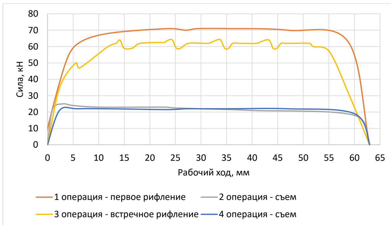
Рисунок 3.18 – График технологической силы, полученный по результатам эксперимента ( Z=0,5 мм, h=1 мм)
