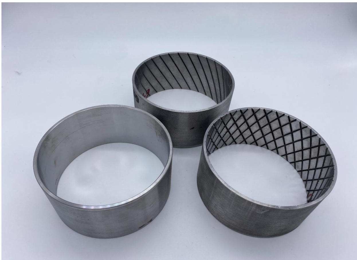
Рисунок 3.24 – Заготовка, полуфабрикат с рифлями одного направления и деталь с сеткой рифлей
