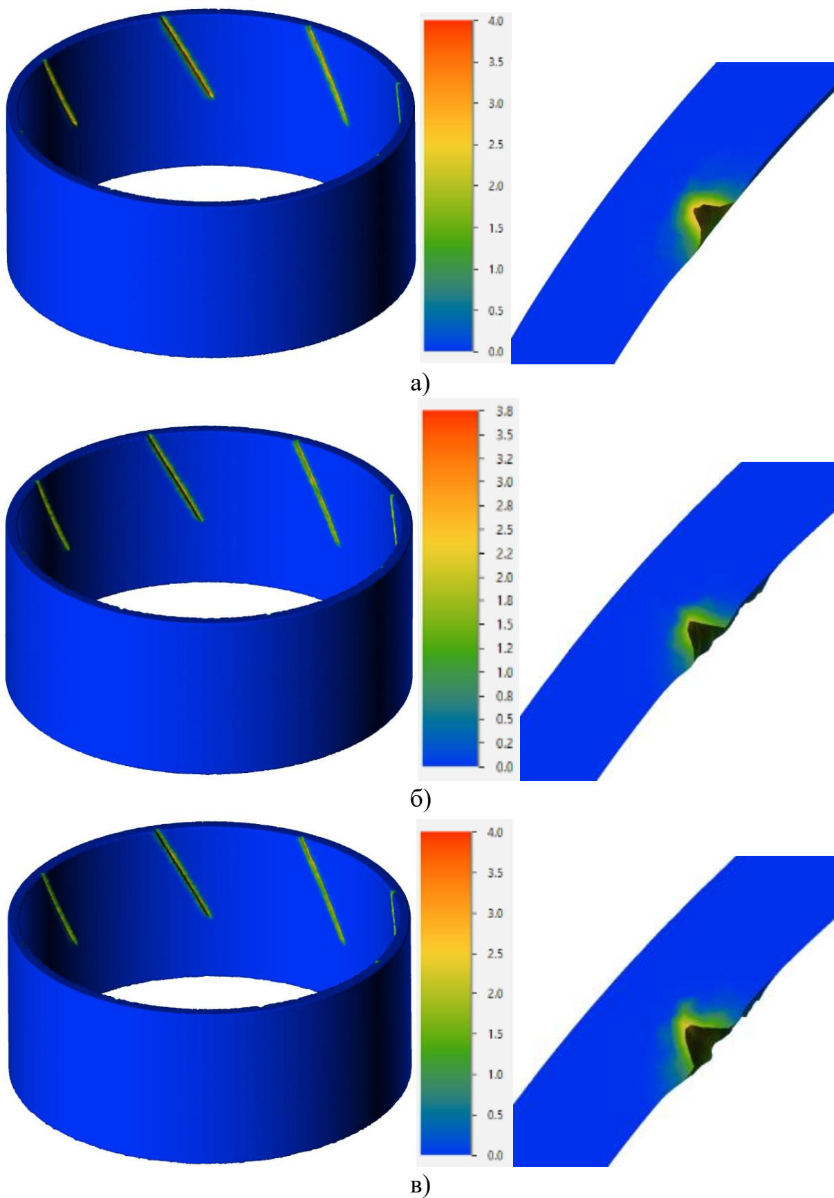
Рисунок 2.18 – Интенсивность деформаций при рифлении на глубину 1 мм: а – при зазоре Z = 0,15 мм; б – при зазоре Z = 0,3 мм; в – при зазоре Z = 0,45 мм
