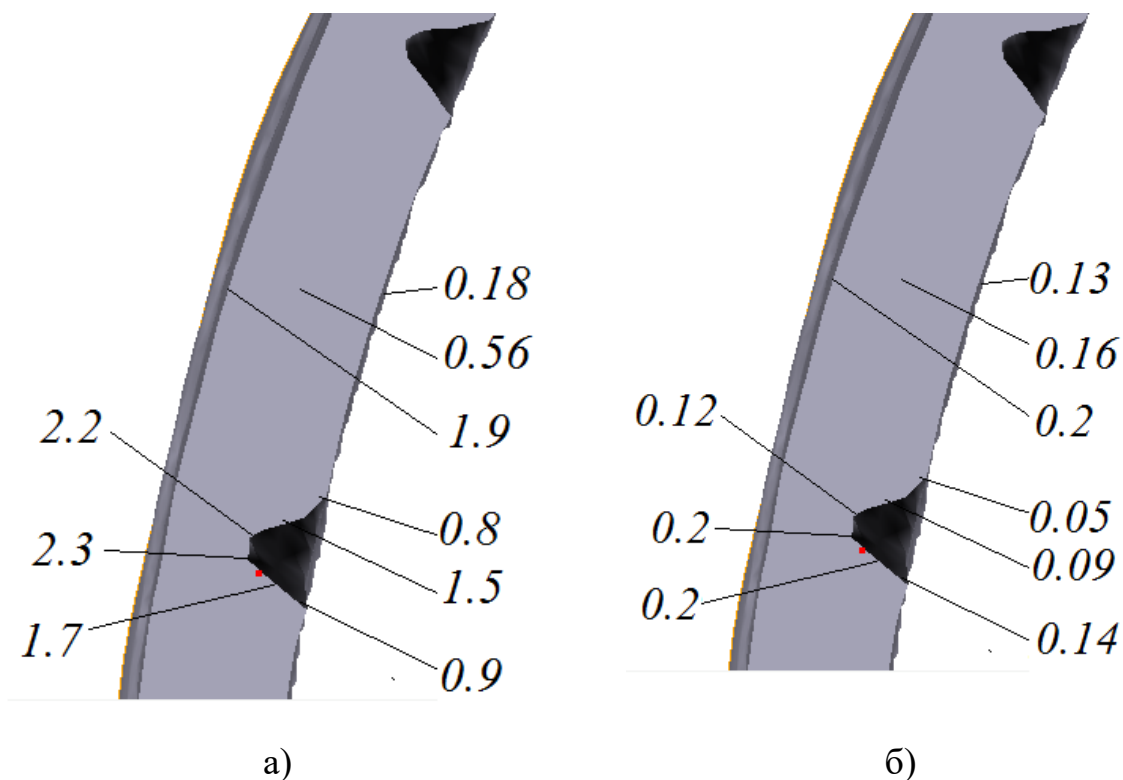
Рисунок 1.12 – Картина, характеризующая изменение интенсивности деформации (а), значения параметра Cockroft_Latham (б) в сечении перпендикулярном к оси заготовки на конечном этапе формирования рифли
