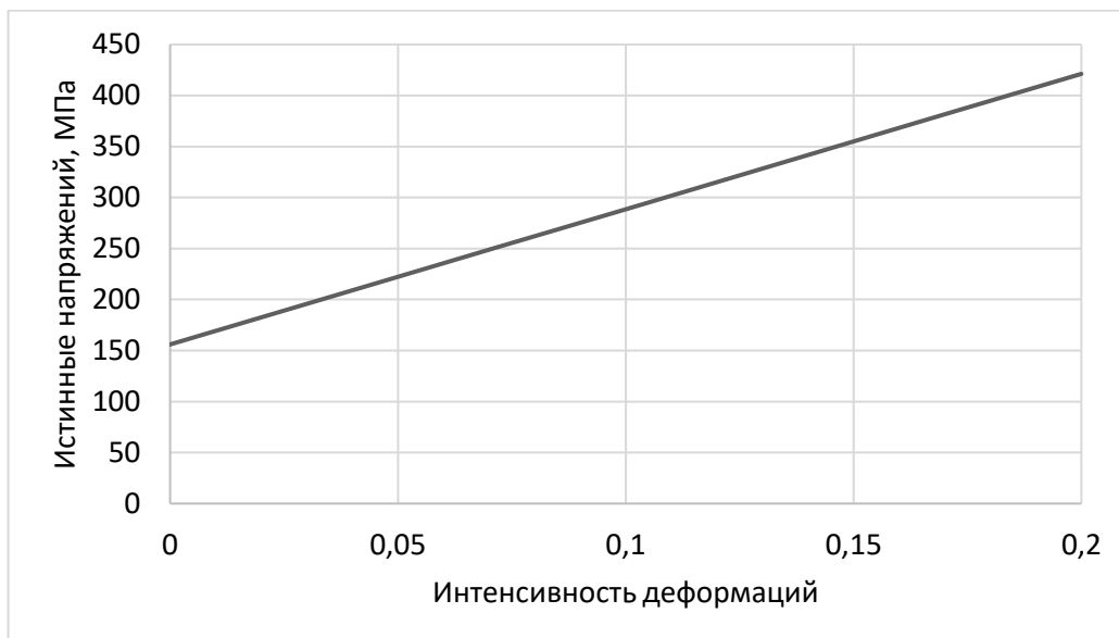
Рисунок 3.12 – Кривая упрочнения для сплава АМг5
