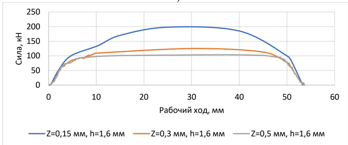
Рисунок 2.11 – График технологической силы рифления для оправки типа III: а – при глубине внедрения 1 мм, б – при глубине внедрения 1,3 мм, в – при глубине внедрения 1,6 мм
