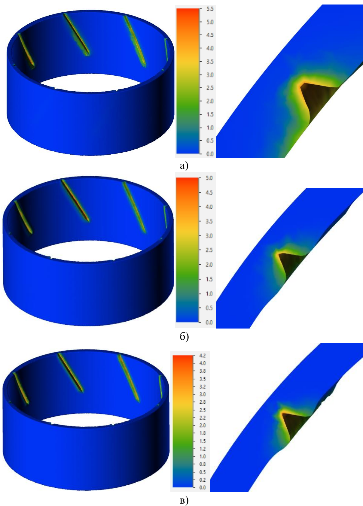
Рисунок 2.20 – Интенсивность деформаций при рифлении на глубину 1,6 мм: а – при зазоре Z = 0,15 мм; б – при зазоре Z = 0,3 мм; в – при зазоре Z = 0,45 мм
