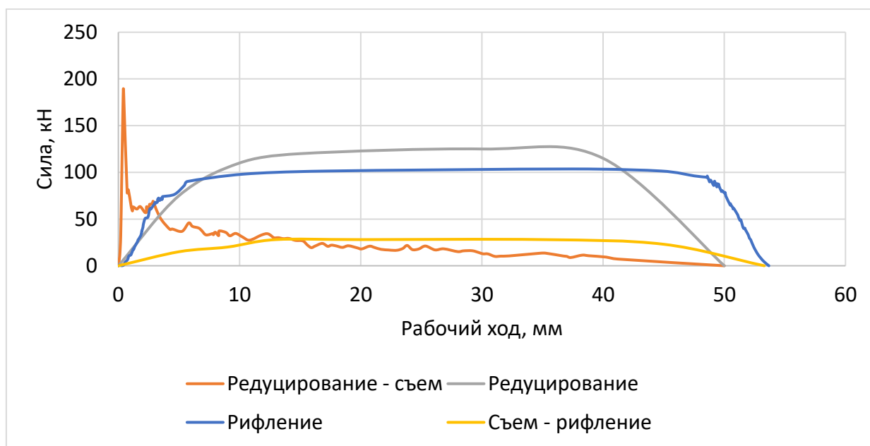
Рисунок 2.33 – График сил
