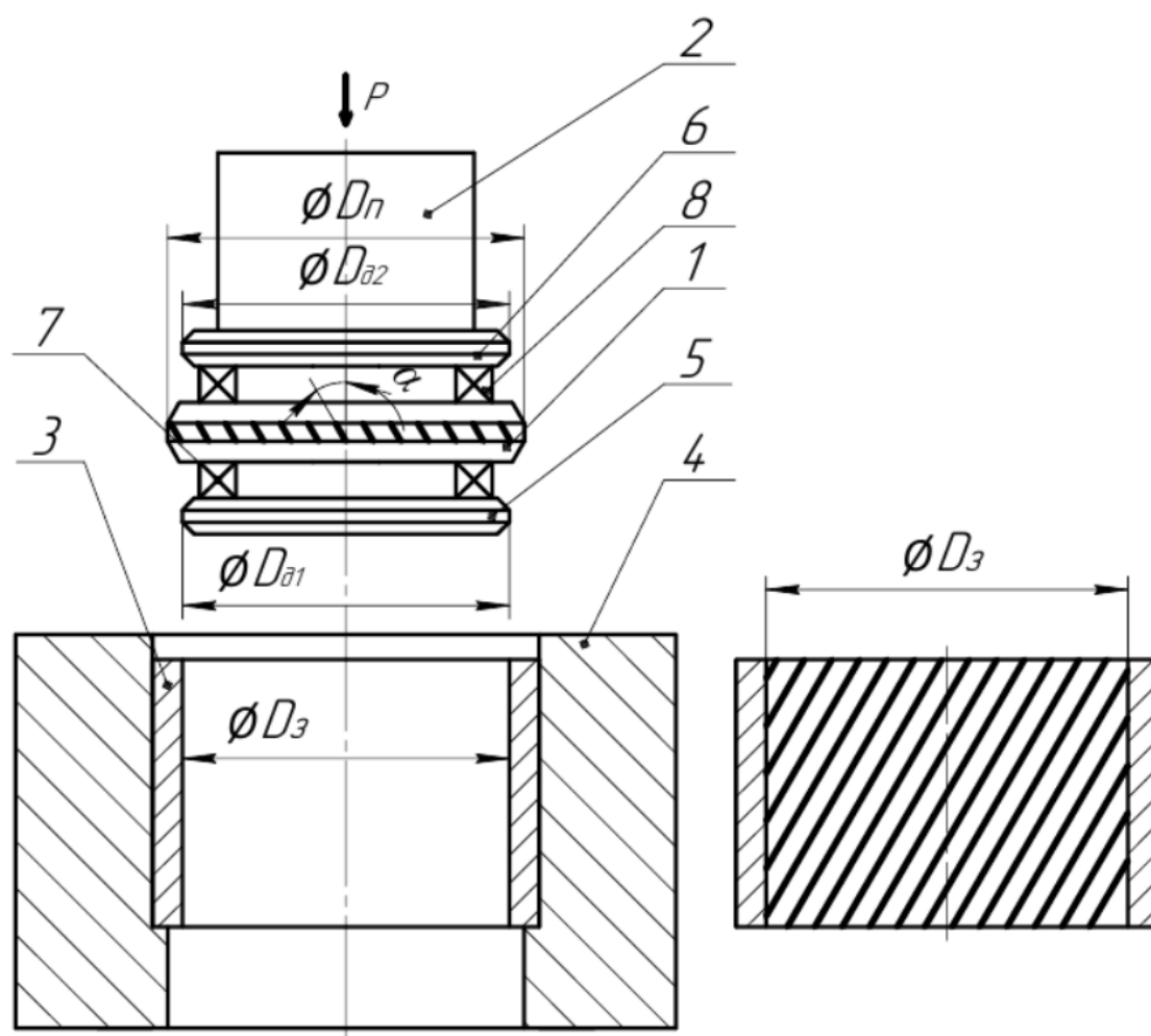
Рисунок 4.5 – Способ изготовления сетки рифлей на внутренней поверхности цилиндрической оболочки
