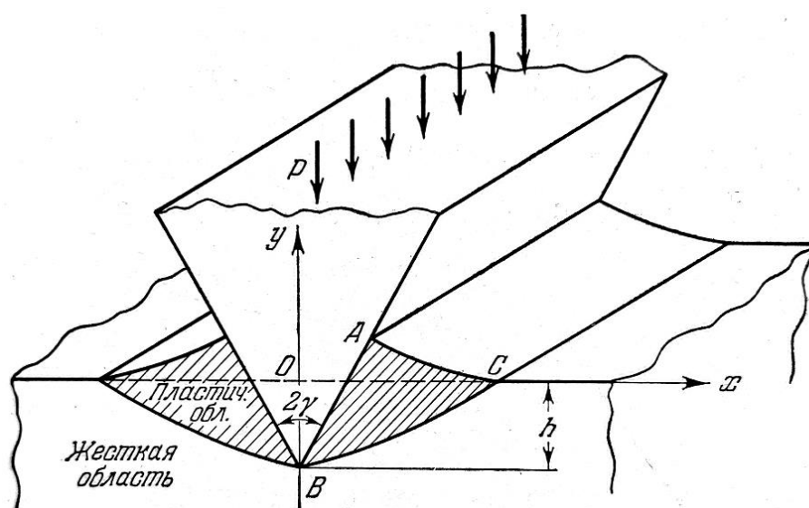
Рисунок 1.7 – Схема деформации при внедрении клина [46]
