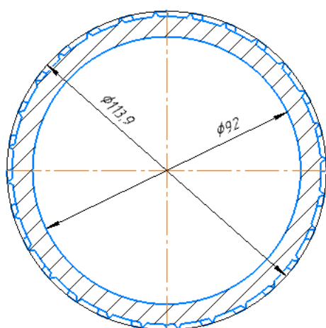
Рисунок 3.5 – Рабочая оправка типа II: а – фотография, б – схема
