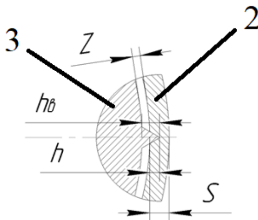
Рисунок 2.6 – Зазор между заготовкой (2) и рабочей оправкой (3)
