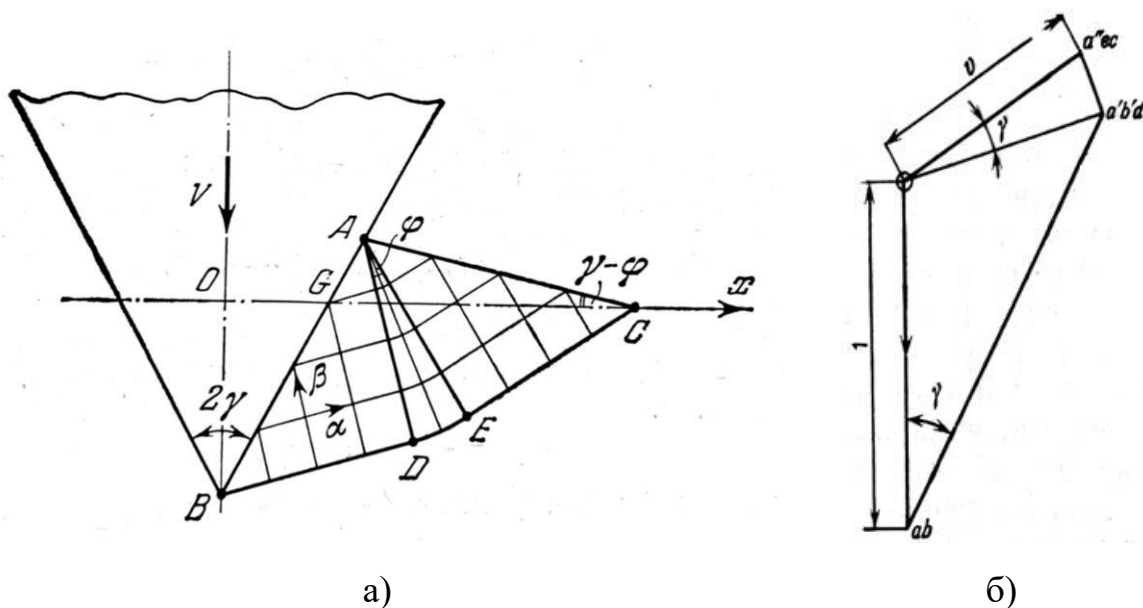
Рисунок 1.8 – Сетка линий скольжения (а), годограф скоростей (б) [46]
