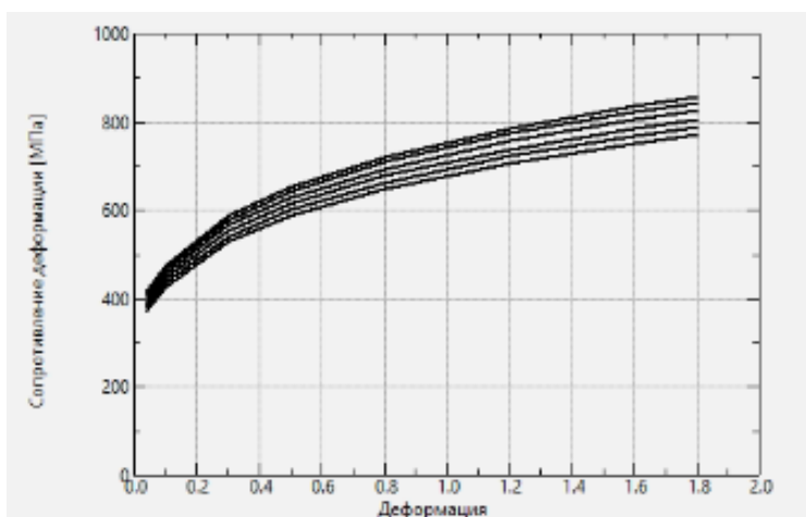
Рисунок 2.5 – Сопротивление деформации материала при разной скорости деформации: 0,01, 0,1, 1, 10, 100, 500 (1/с)
