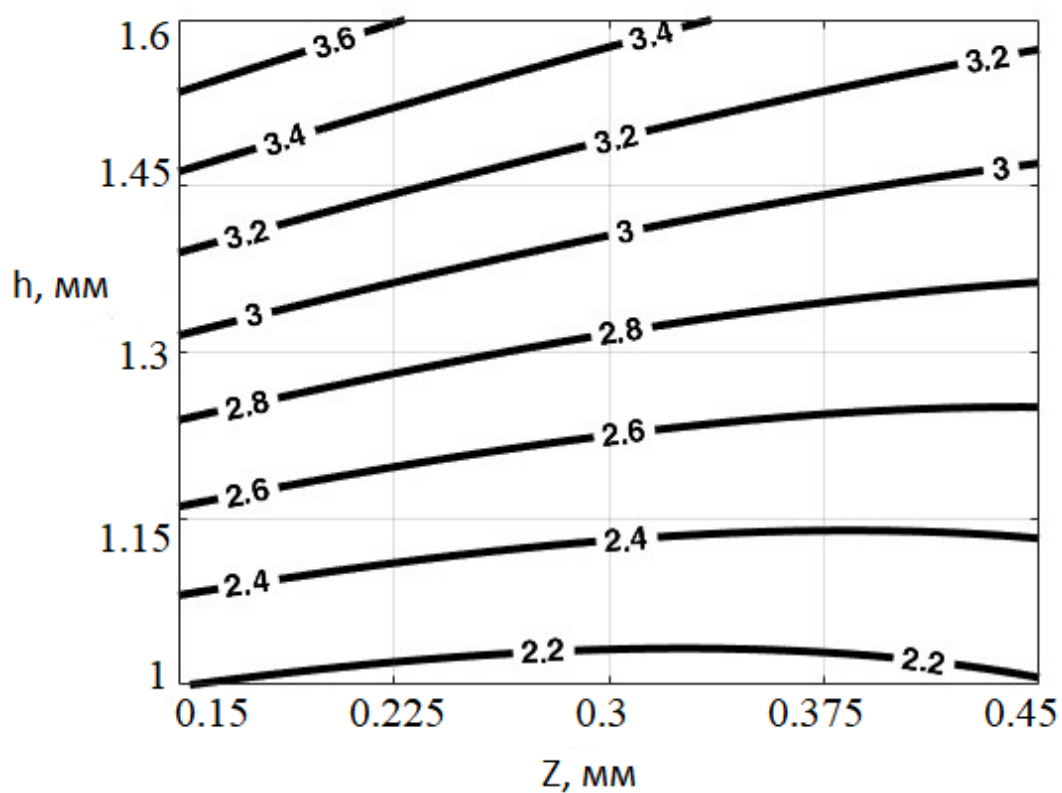
Рисунок 2.31 – Зависимость интенсивности деформаций ( \epsilon_i ) от величин ( Z, h )
