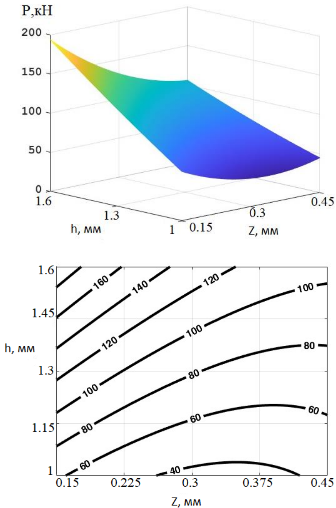
Рисунок 2.12 – Зависимость максимальной технологической силы рифления ( P ) от величин ( Z , h )
