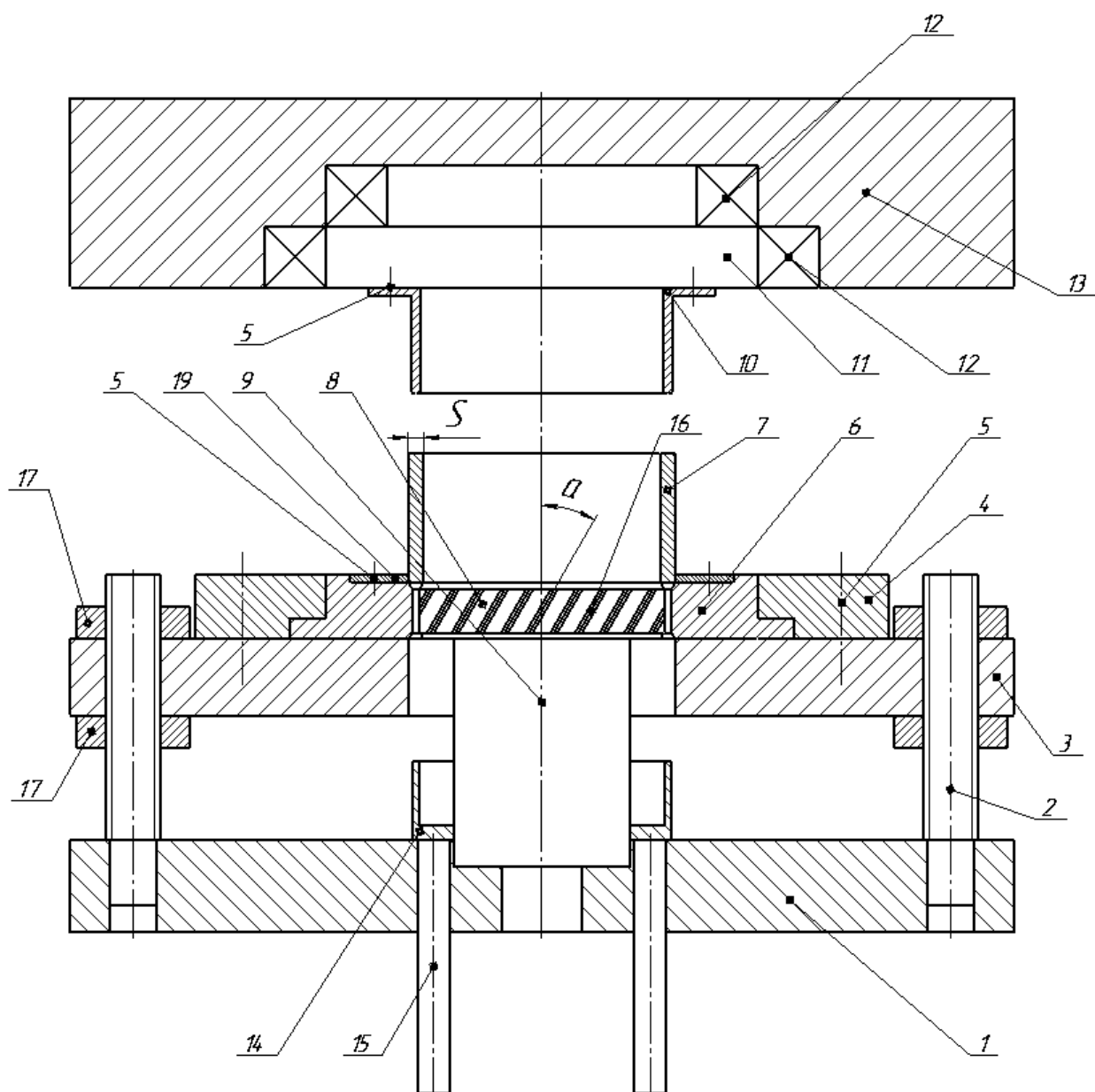
Рисунок 4.9 – Конструкция нового устройства для одновременного рифления и наружной поверхности, и внутренней
