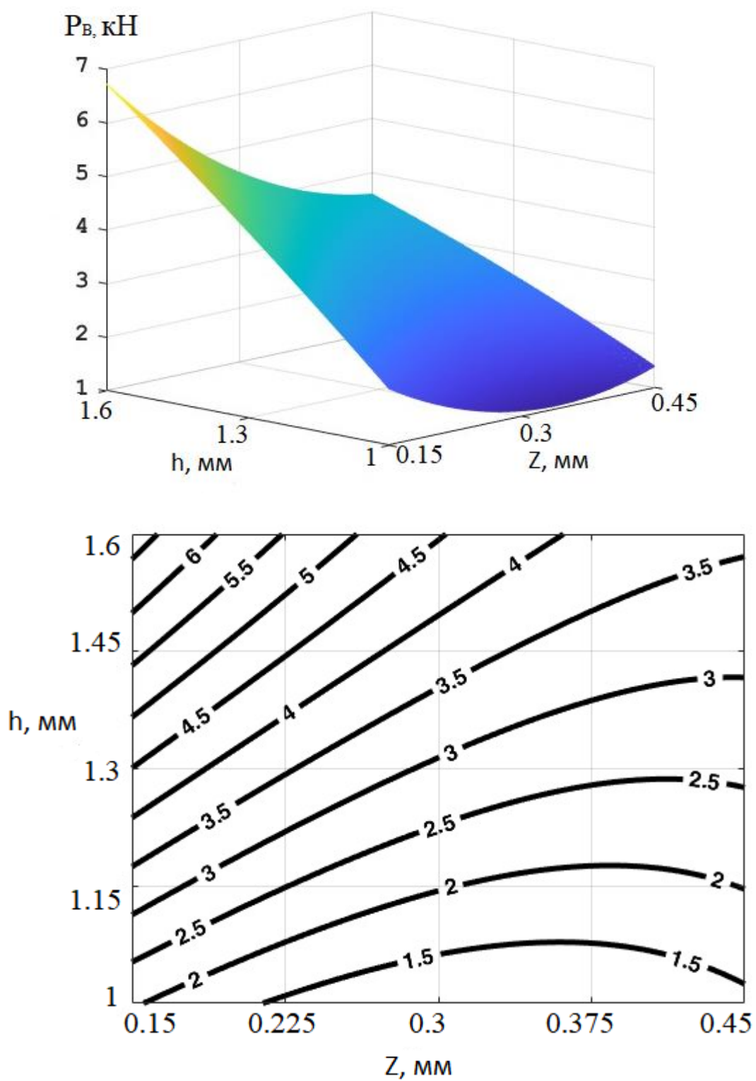
Рисунок 2.13 – Зависимость силы рифления на один выступ ( P_B ) от величин ( Z , h )
