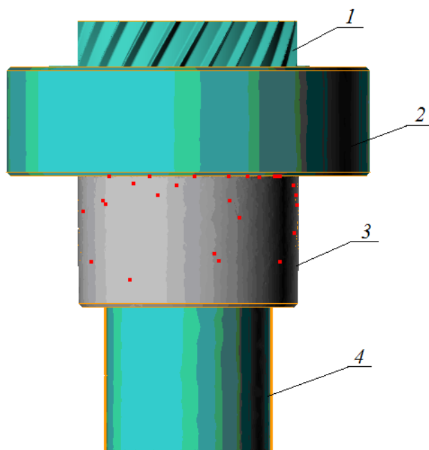
Рисунок 1.13 – Схема процесса съема заготовки с профильного пуансона: 1 – пуансон; 2 – съемник; 3 – заготовка; 4 – упор
