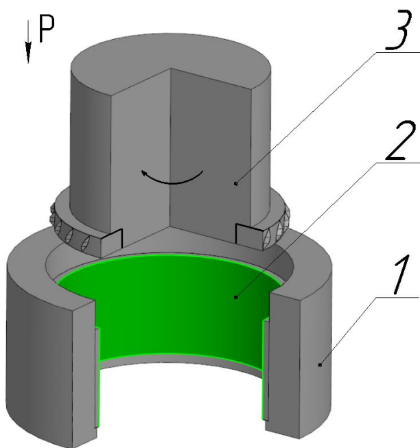
Рисунок 2.1 – Схема процесса изготовления рифлей на внутренней поверхности металлической оболочки: 1 – контейнер, 2 – цилиндрическая оболочка, 3 – инструментальный стержень с рабочей оправкой
