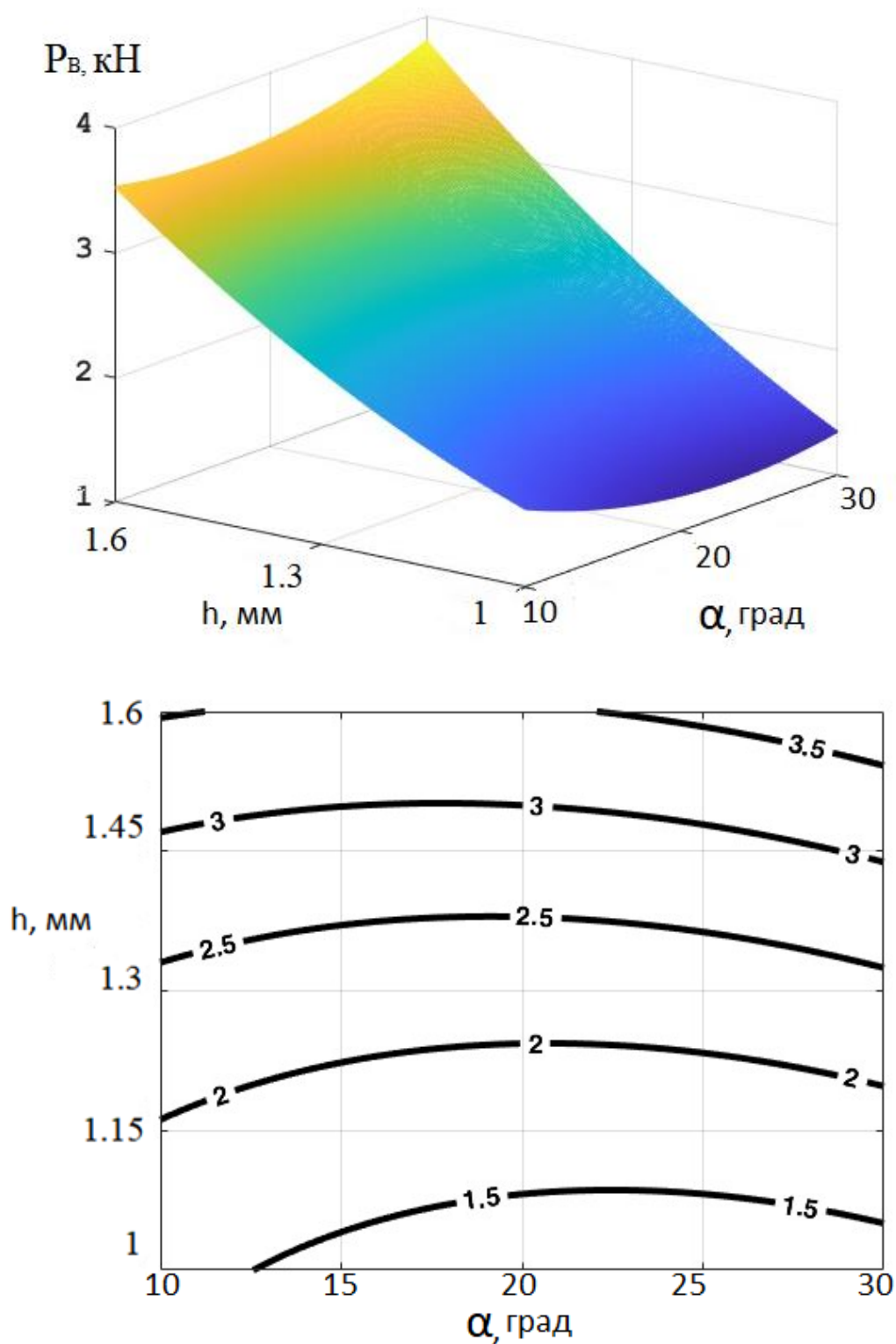
Рисунок 2.17 – Зависимость силы rifления на один выступ ( P_B ) от величин ( \alpha , h ) при rifлении с зазором Z=0,45 мм
