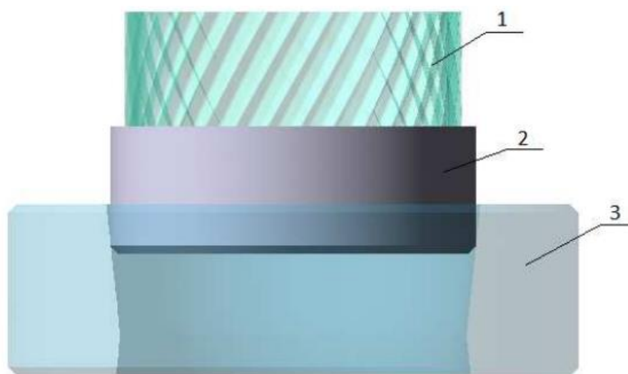
Рисунок 1.11 – Схема процесса редуцирования [22]: 1 – пуансон; 2 – заготовка; 3 – матрица
