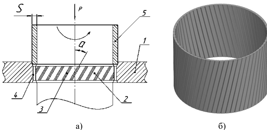
Рисунок 4.7 – Первая операция одновременного рифления и наружной поверхности, и внутренней: а – схема операции, б – получаемый полуфабрикат
