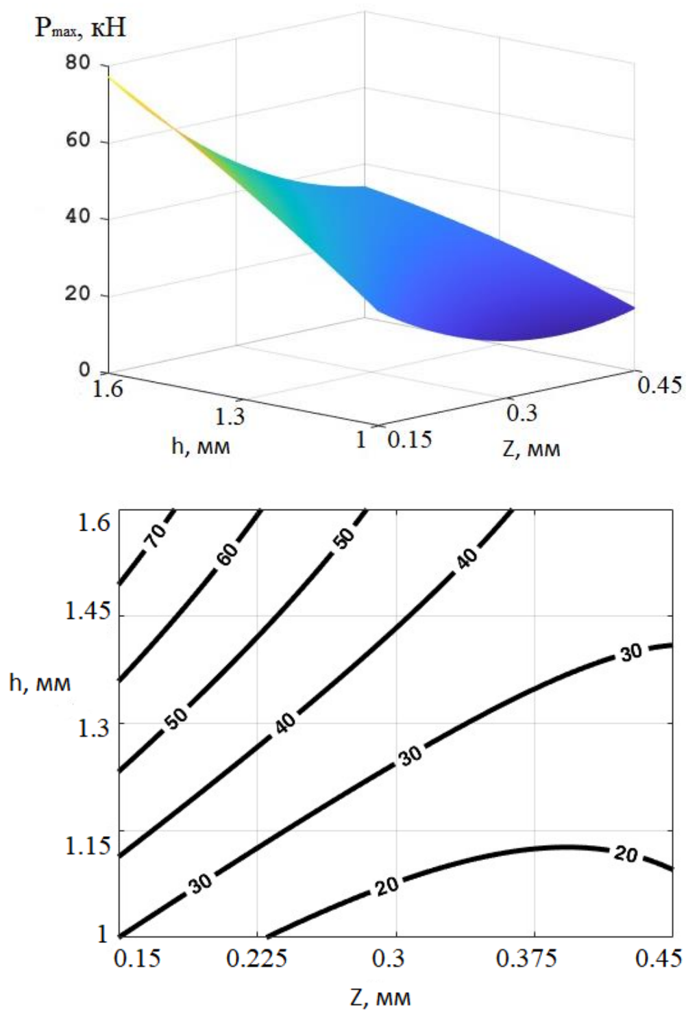
Рисунок 2.14 – Зависимость максимальной технологической силы съёма ( P_{max} ) от величин ( Z , h )
