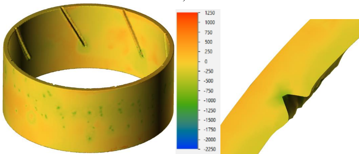
Рисунок 2.22 – Средние напряжения при рифлении на глубину 1,3 мм: а – при зазоре Z = 0,15 мм; б – при зазоре Z = 0,3 мм; в – при зазоре Z = 0,45 мм
