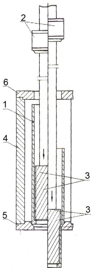
Рисунок 1.6 – Схема для формирования рифлей редуцированием: 1 – заготовка; 2 – пуансон; 3 – спиральный выступ; 4 – корпус штамповой оснастки; 5 – калибровочная матрица; 6 – кольцевой съемник
