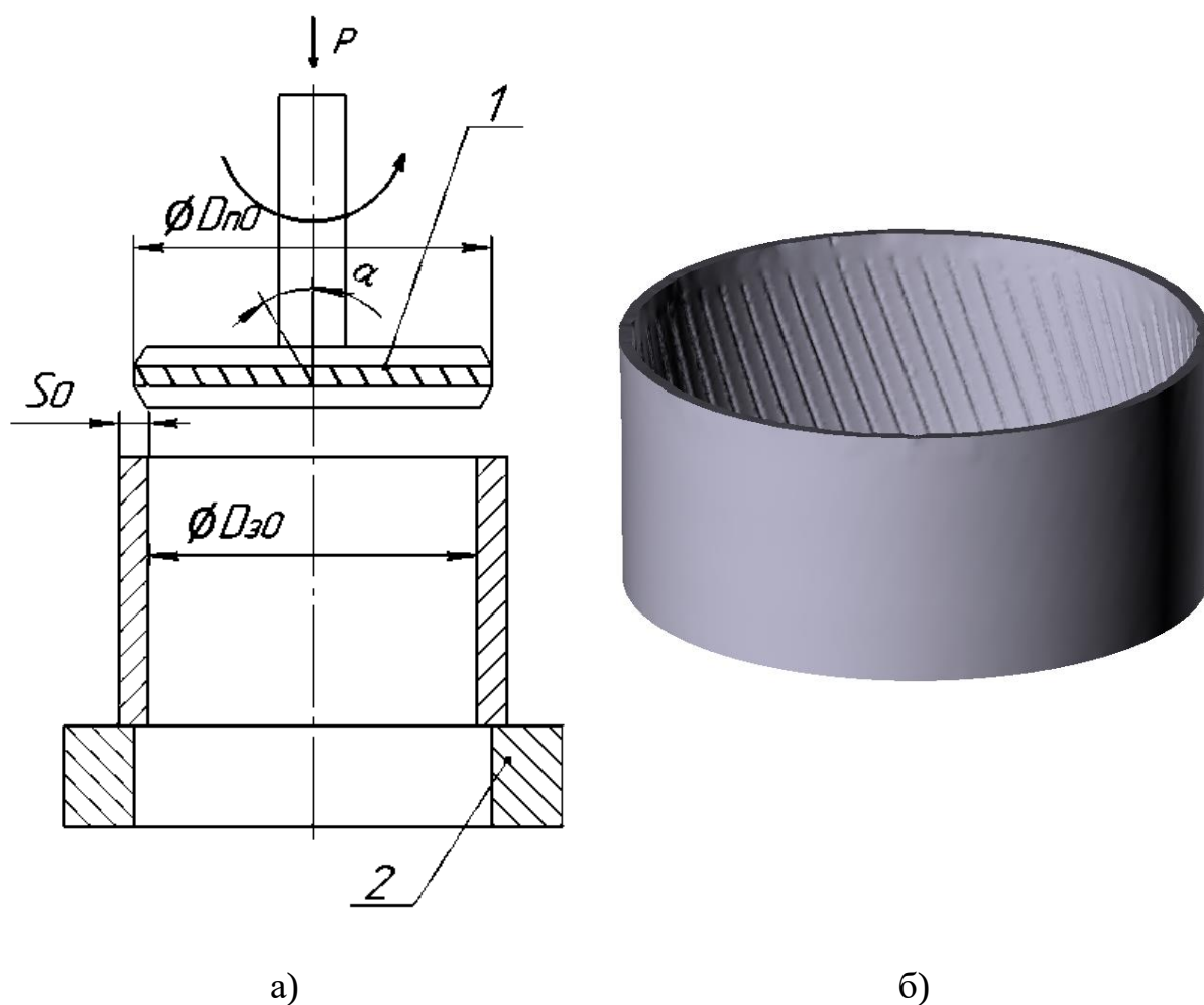
Рисунок 4.2 – Рифление с процессом одновременной раздачи на первой операции: а – схема процесса, б – полуфабрикат
