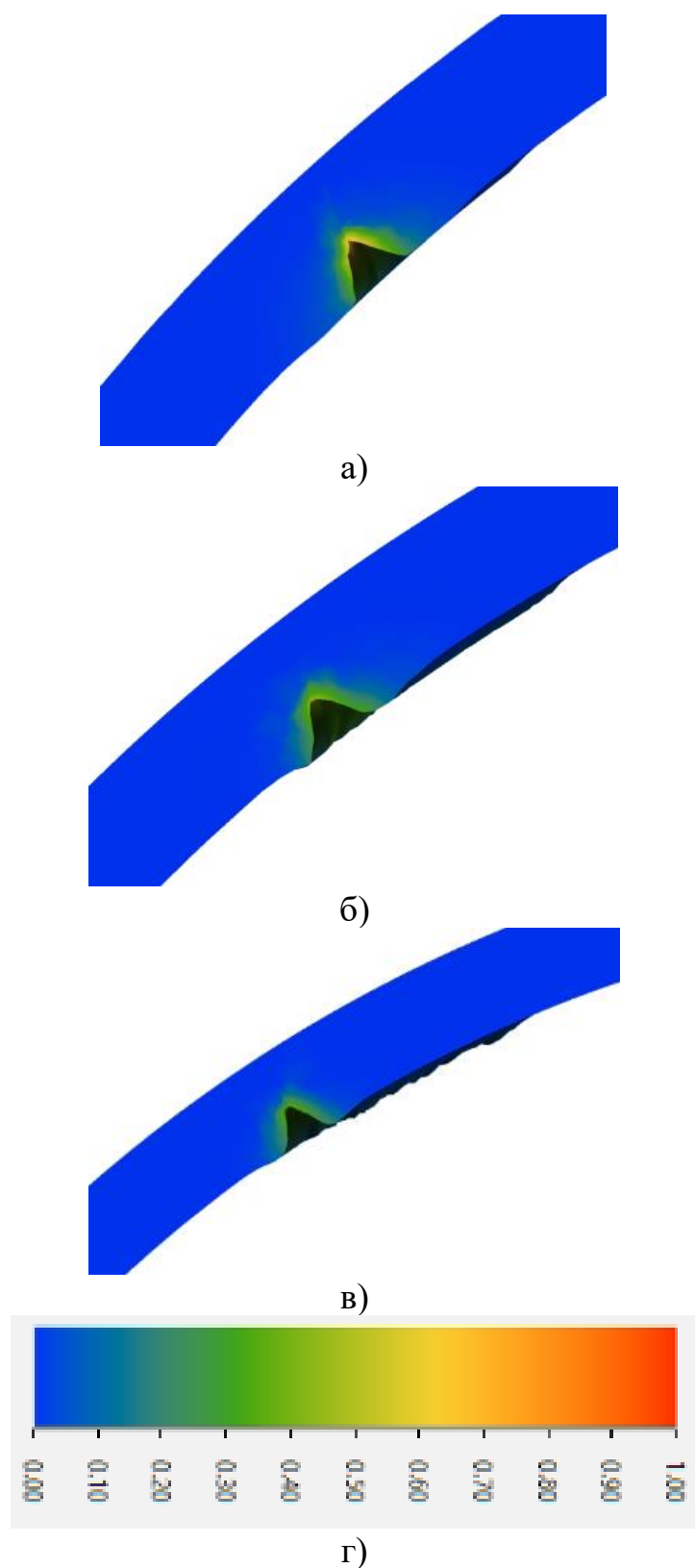
Рисунок 2.26 – Повреждаемость материала при рифлении оправкой типа III на глубину 1,3 мм: а – при зазоре Z = 0,15 мм; б – при зазоре Z = 0,3 мм; в – при зазоре Z = 0,45 мм; г – шкала
