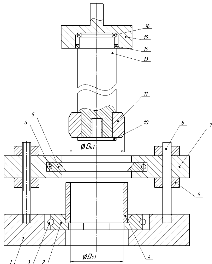
Рисунок 4.4 – Схема устройства для реализации способа рифления с раздачей
