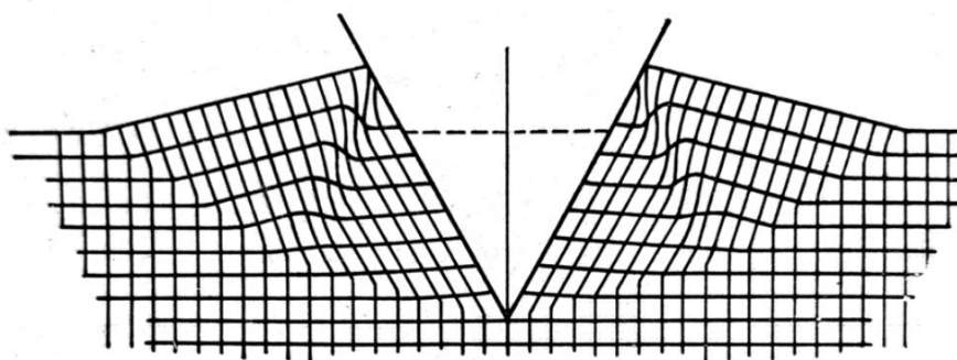
Рисунок 1.9 – Искажение первоначальной квадратной сетки [46]
