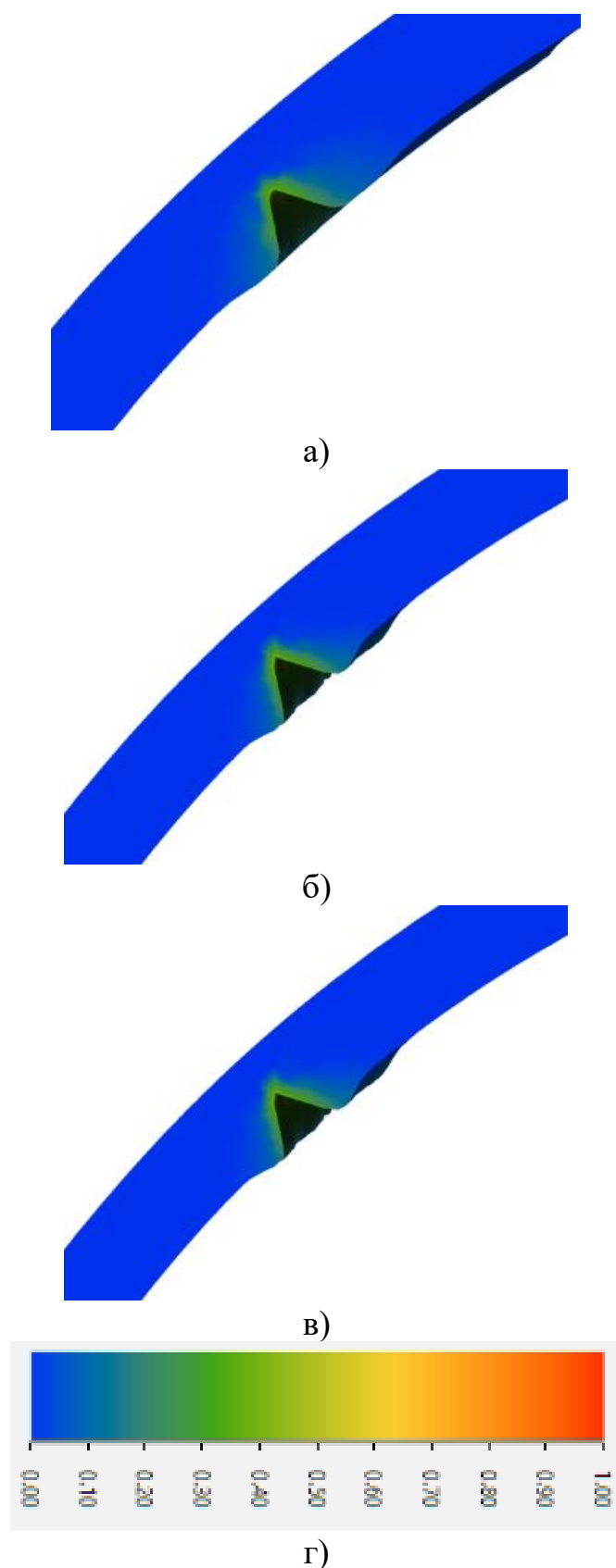
Рисунок 2.27 – Повреждаемость материала при рифлении оправкой типа III на глубину 1,6 мм: а – при зазоре Z = 0,15 мм; б – при зазоре Z = 0,3 мм; в – при зазоре Z = 0,45 мм; г – шкала
