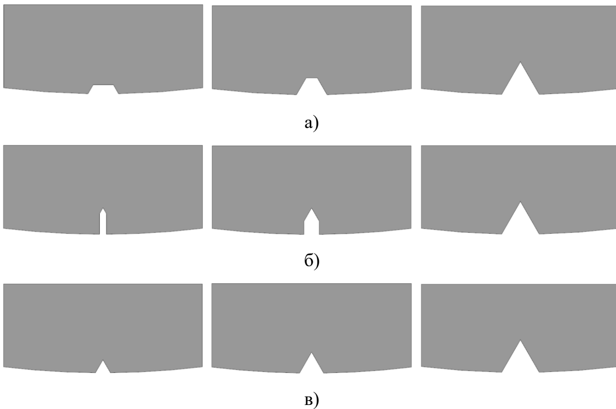
а) б) в) Рисунок 2.8 – Стадии внедрения выступов рабочих оправок в заготовку, при разных типах заходных частей: а – тип I, б – тип II, в – тип III
