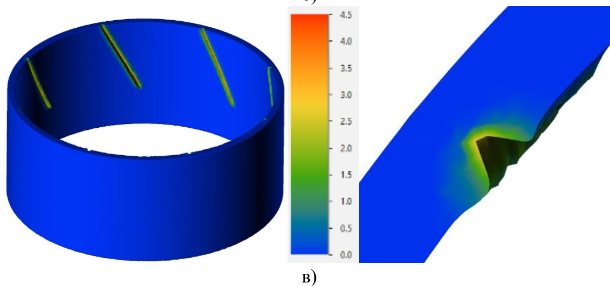
Рисунок 2.19 – Интенсивность деформаций на глубину 1,3 мм: а при зазоре Z = 0,15 мм; б – при зазоре Z = 0,3 мм; в – при зазоре Z = 0,45 мм
