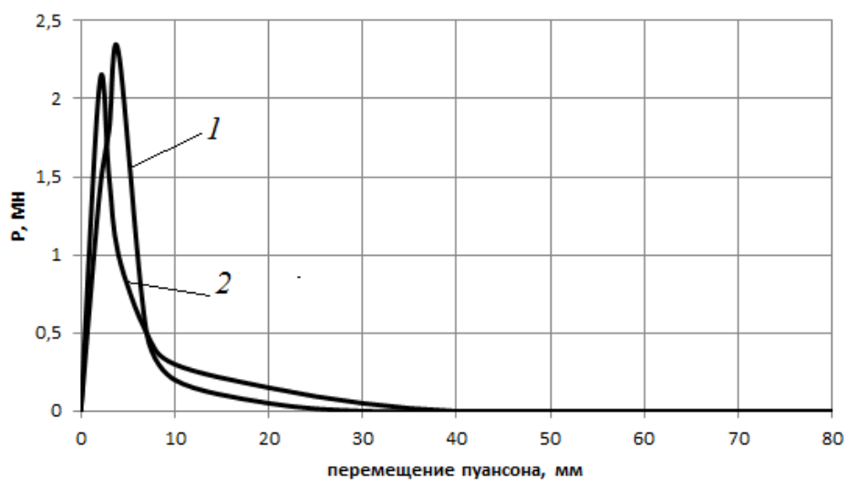
Рисунок 1.16 – Сила съема полуфабриката с рифленого пуансона с левыми рифлями: 1 – экспериментальная кривая; 2 – теоретическая кривая
