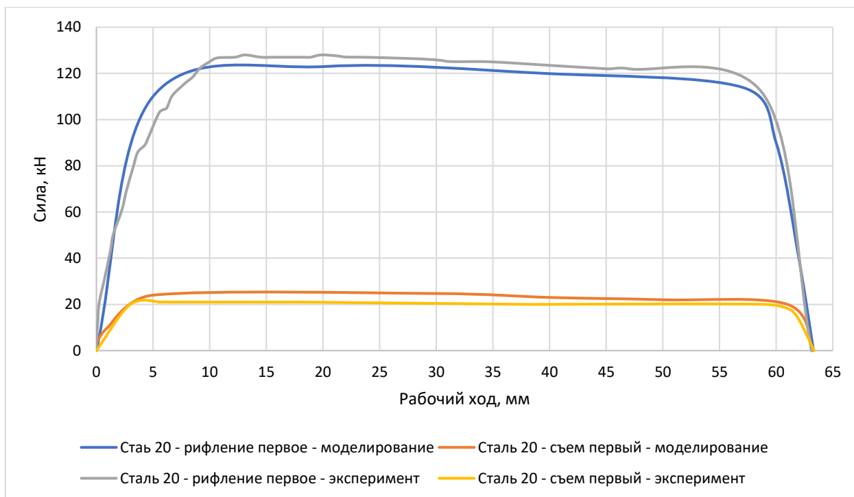
Рисунок 3.25 – График силы рифления
