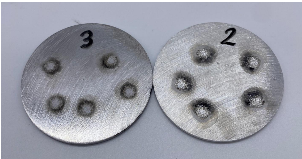
Рисунок 3.9 – Образцы, подверженные спектрометрии: образец слева – сталь 20, образец справа – АМг5
