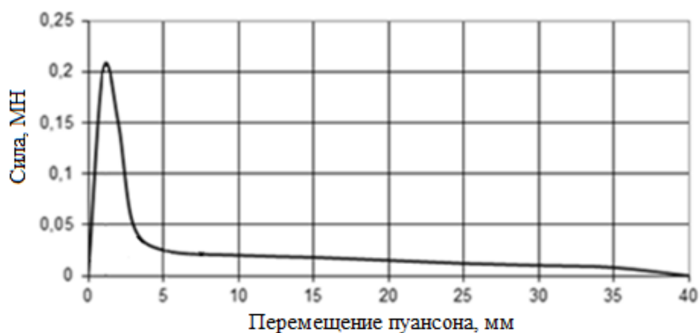
Рисунок 1.14 – Сила процесса съема заготовки после первой операции редуцирования
