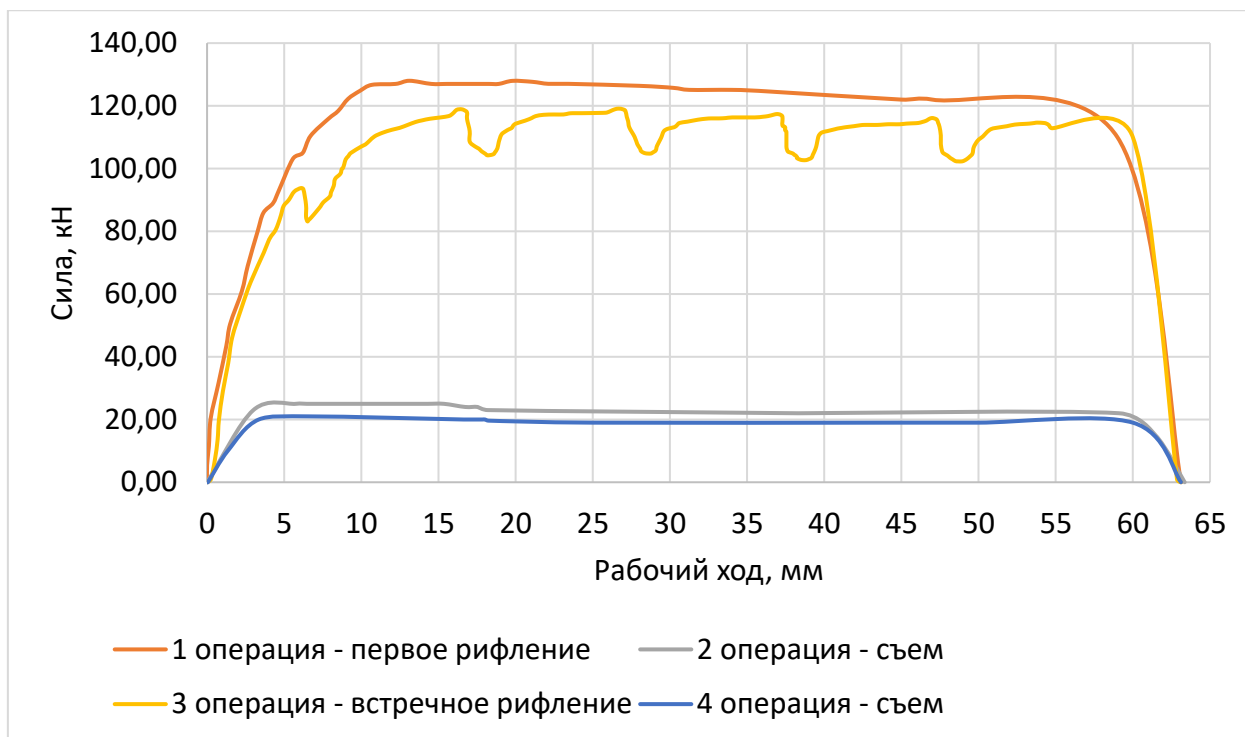
Рисунок 3.23 – График технологической силы при рифлении стального образца при эксперименте №1 ( Z=0,5 мм, h=1 мм)
