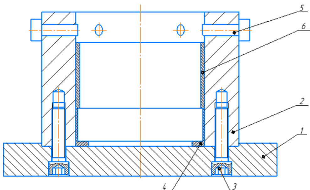
Рисунок 3.2 – Схема экспериментального штампа (нижняя часть)
