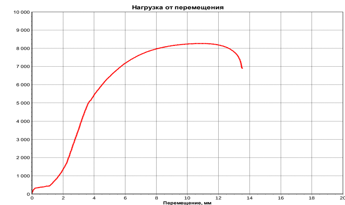
Рисунок 3.11 – Кривая «Нагрузка-перемещение» для образцов из алюминиевого сплава АМг5
