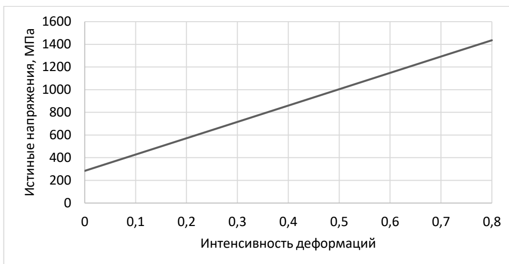
Рисунок 3.13 – Кривая упрочнения для стали 20
