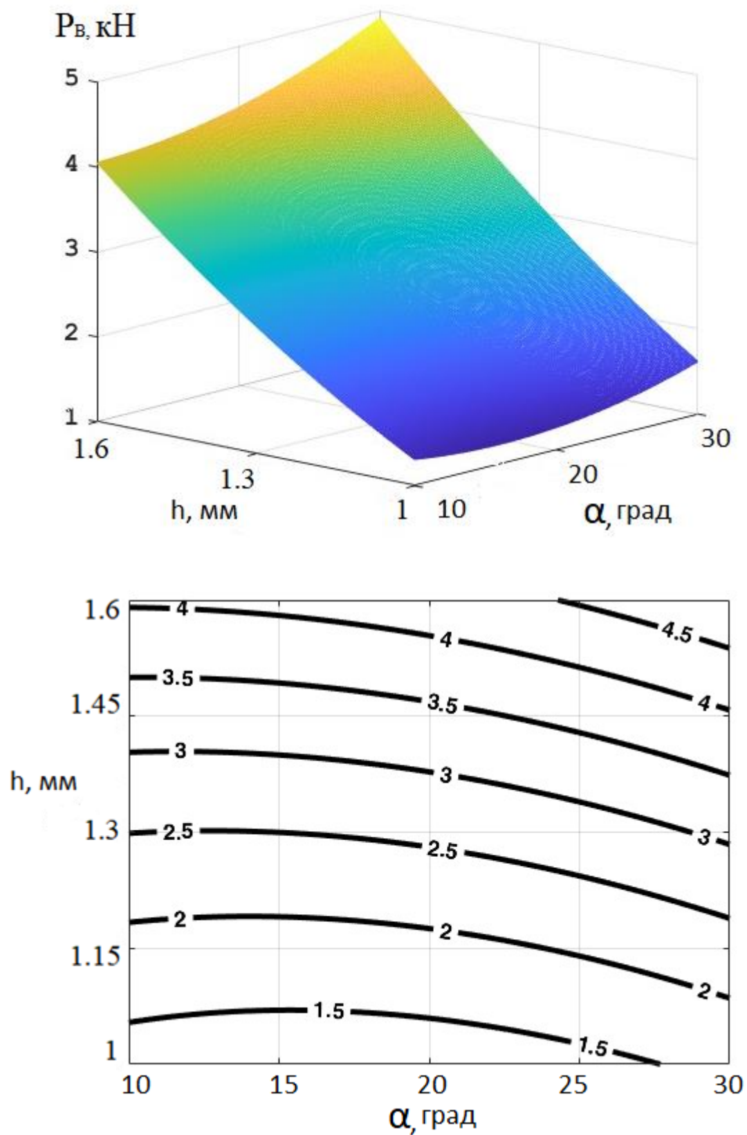
Рисунок 2.16 – Зависимость силы рифления на один выступ ( P_B ) от величин ( \alpha , h ) при рифлении с зазором Z=0,3 мм
