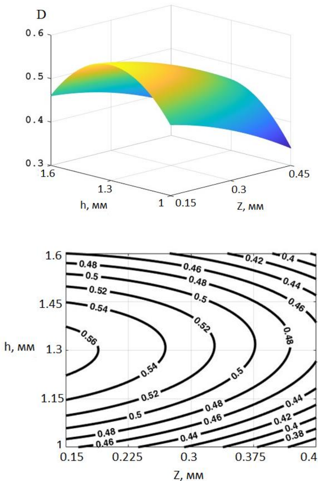
Рисунок 2.30 – Зависимость максимального значения повреждаемости ( D ) от величин ( Z, h )
