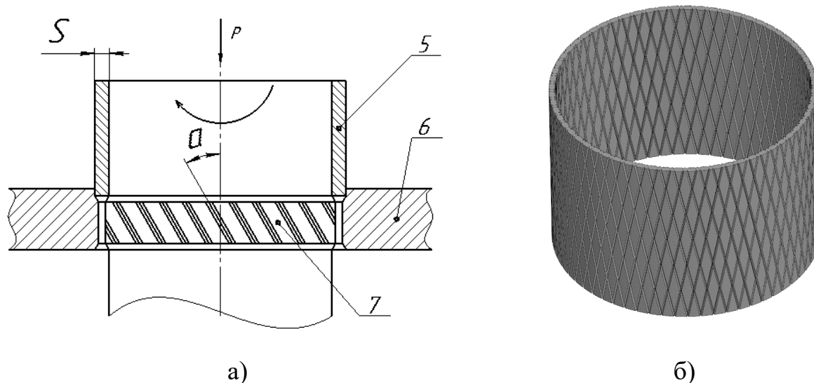
Рисунок 4.8 – Вторая операция одновременного рифления наружной и внутренней поверхностей: а – схема операции, б – получаемый полуфабрикат
